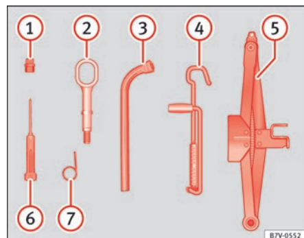
Fig. 198 Componentes del juego de herramientas de a bordo.
