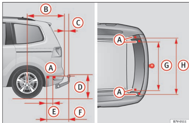
Fig. 157 Cotas y puntos de fijación para instalar posteriormente un enganche para remolque.
