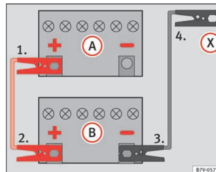
Fig. 216 Esquema de conexión de los cables de emergencia cuando un vehículo sin sistema Start-Stop suministra la corriente: batería descargada (A) y batería que suministra la corriente (B).
