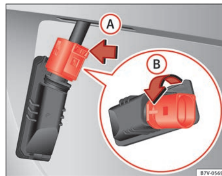
Fig. 214 Luz de la matrícula: Desmontar el portalámparas.
