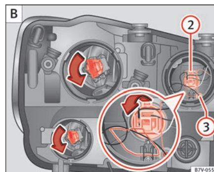
Fig. 204 Faro izquierdo
