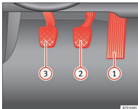
Fig. 128 Pedales en vehículos con cambio manual: ① acelerador; ② freno; ③ embrague.
