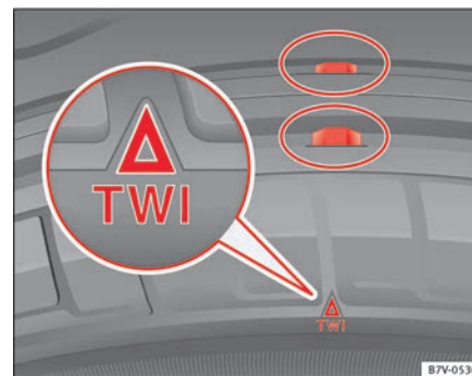
Fig. 177 Perfil del neumático: indicadores de desgaste.
