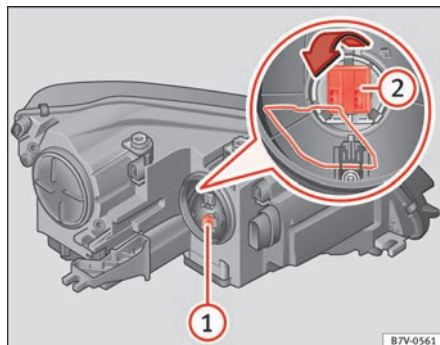
Fig. 206 Portalámparas del intermitente ① y luz para curvas ②.
