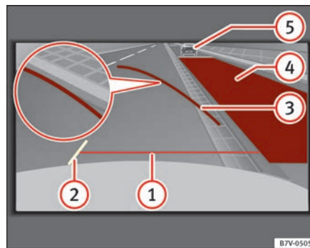
Fig. 149 Pantalla: líneas y superficies de orientación del espacio detrás del vehículo.
