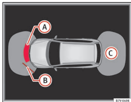
Fig. 142 Indicación del OPS en pantalla: (A) se ha detectado un obstáculo en la zona de colisión. (B) se ha detectado un obstáculo en el segmento. (C) zona registrada detrás del vehículo.
