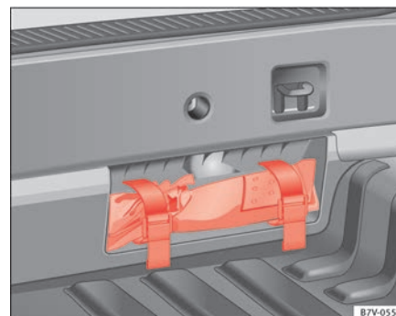
Fig. 197 En el maletero, visto desde el interior del vehículo: Herramientas de a bordo en una cavidad situada en la zona del portacierres.
