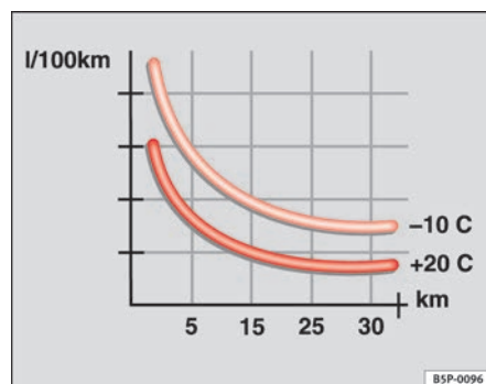
Fig. 155 Consumo de combustible (l/100 km) a diferente temperatura ambiental.
