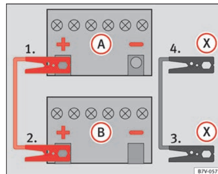
Fig. 217 Esquema de conexión de los cables de emergencia cuando un vehículo con sistema Start-Stop suministra la corriente: batería descargada (A) y batería que suministra la corriente (B).
