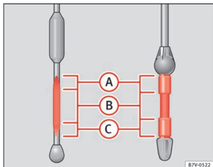
Fig. 168 Varilla de medición con marcas para el nivel del aceite.
