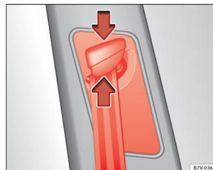
Fig. 15 Junto a los asientos delanteros: regulador de la altura del cinturón.
