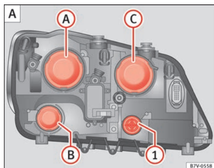
Fig. 203 En el vano motor: Revestimientos en el faro izquierdo. (A) luces de cruce, (B) luz diurna y (C) luz de carretera y luz de posición.
