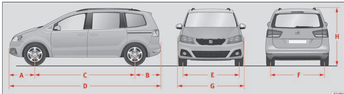
Fig. 257 Dimensiones
