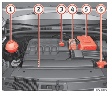
Fig. 242 Figura orientativa de la posición de los elementos.
