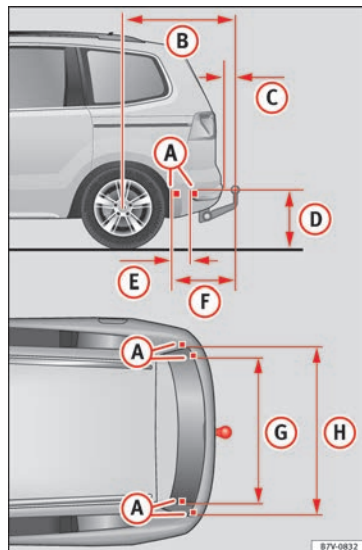
Fig. 233 Cotas y puntos de fijación para instalar posteriormente un enganche para remolque.
