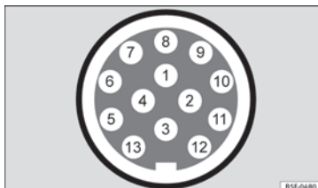
Fig. 232 Representación esquemática: asignación de los pines de la toma de corriente del remolque.
