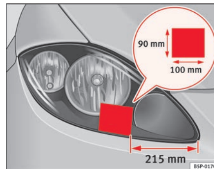
Fig. 154 Faro derecho
