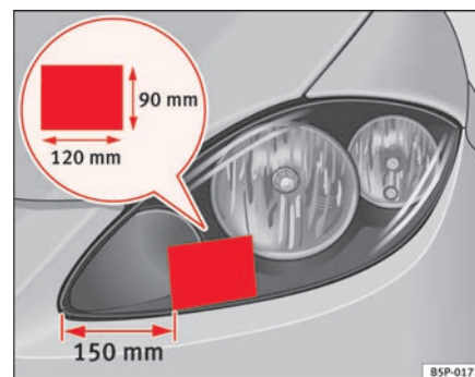
Fig. 155 Faro izquierdo ▶
