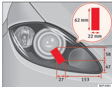
Fig. 158 Faro derecho
