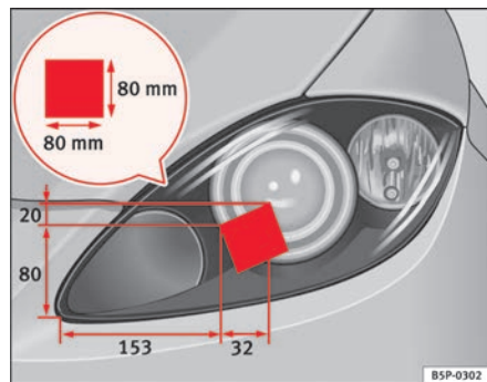
Fig. 159 Faro izquierdo
