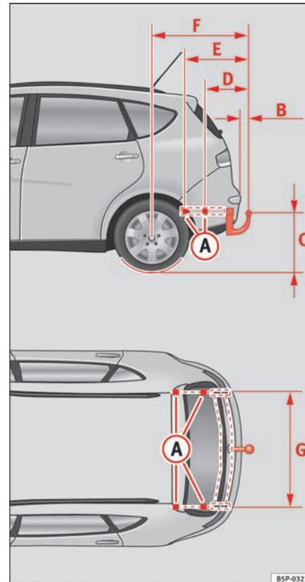
Fig. 160 Puntos de fijación del dispositivo de remolque
