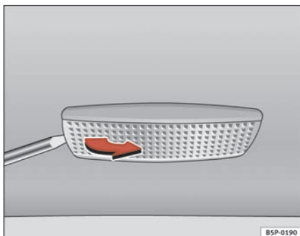
Fig. 202 Desmontaje luz del parasol
