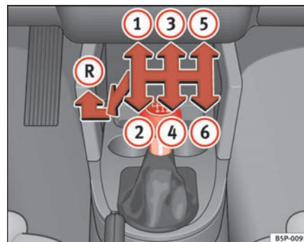
Fig. 139 Detalle de la consola central: esquema de un cambio manual de 6 marchas
