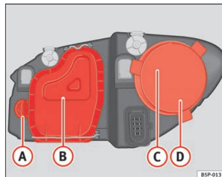
Fig. 185 Lámparas del faro principal
