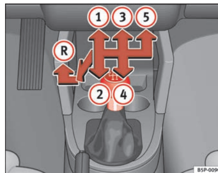
Fig. 138 Detalle de la consola central: esquema de un cambio manual de 5 marchas
