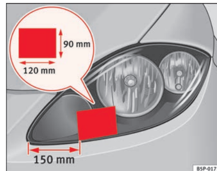
Fig. 157 Faro izquierdo
