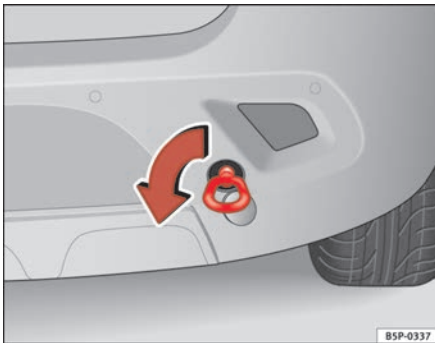
Fig. 208 Argolla de remolque trasera para vehículos con tracción total
