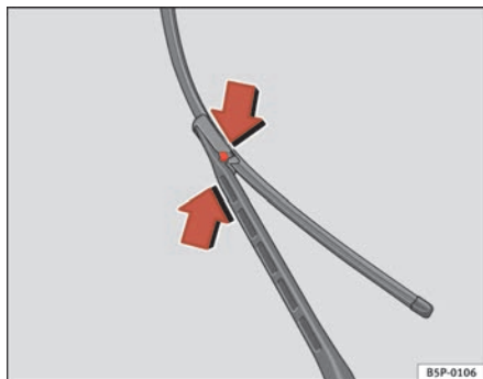
Fig. 170 Cambio de las escobillas del limpiaparabrisas
