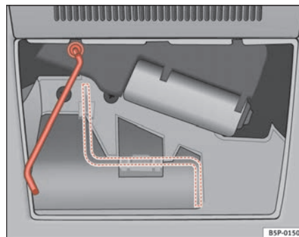
Fig. 71 Manivela cierre de emergencia
