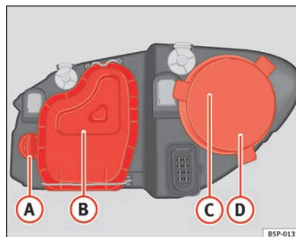
Fig. 180 Lámparas del fero principal
