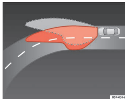
Fig. 75 Iluminación de la curva con faros autodireccionables
