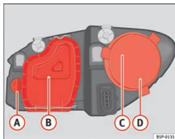
Fig. 179 Lámparas del faro principal
