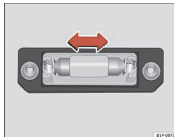
Fig. 195 Luz matrícula
