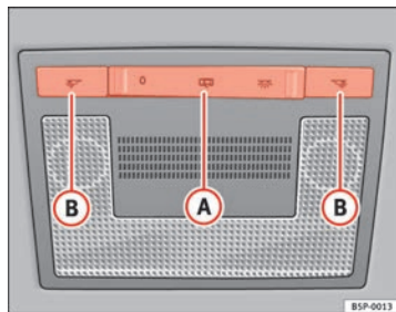
Fig. 79 Revestimiento interior del techo: iluminación delantera del habitáculo
