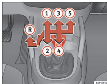
Fig. 139 Detalle de la consola central: esquema de un cambio manual de 5 marchas
