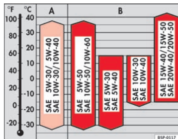
Fig. 157 Tipos de aceite de acuerdo a la temperatura
