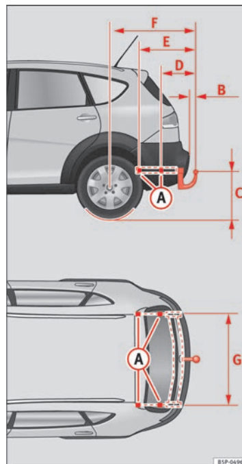
Fig. 153 Puntos de fijación del dispositivo de remolque
