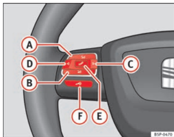
Fig. 56 Mandos en el volante
