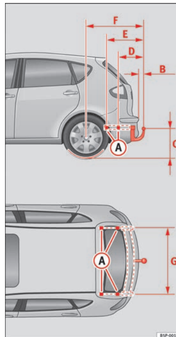
Fig. 155 Puntos de fijación del dispositivo de remolque
