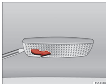
Fig. 199 Desmontaje luz del parasol
