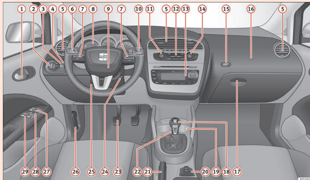
Fig. 33 Tablero de instrumentos
