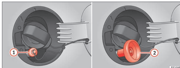
Fig. 157 Tapa del depósito abierta con boca de carga de GLP y adaptador.
