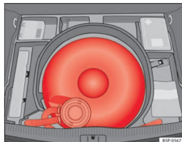
Fig. 158 Depósito de GLP en la cavidad de la rueda de repuesto.
