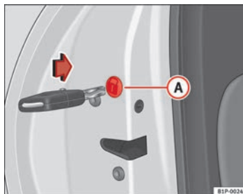
Fig. 60 Cierre de emergencia de las puertas
