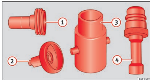
Fig. 159 Cuadro general de los adaptadores para la boca de carga de GLP.
