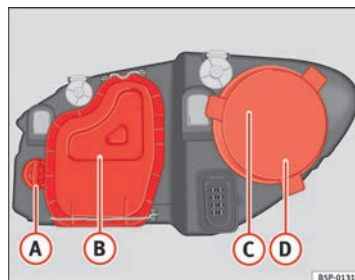
Fig. 181 Lámparas del faro principal
