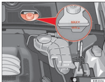
Fig. 187 Compartimento del motor: marcas en el depósito del líquido de frenos
