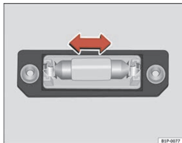
Fig. 240 Luz matrícula
