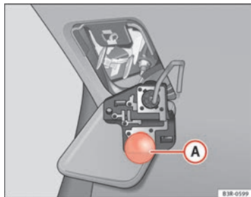
Fig. 218 Ubicación de la lámpara de incandescencia en el portalámparas. Ejemplo: Luces posteriores en el portón del maletero
