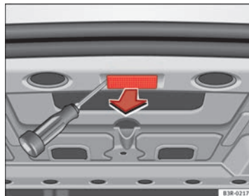
Fig. 220 Luz maletero
