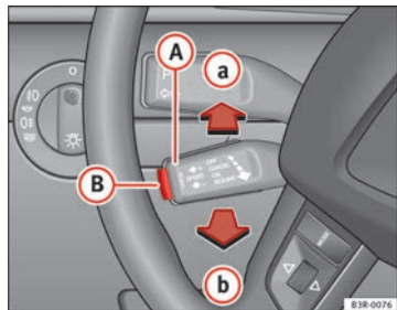
Fig. 141 Mandos del regulador de velocidad
