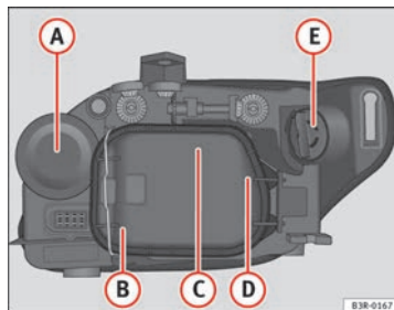
Fig. 189 Lámparas del halógeno
