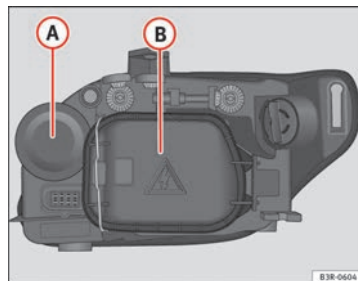
Fig. 201 Lámparas del faro Bi-Xenón AFS
