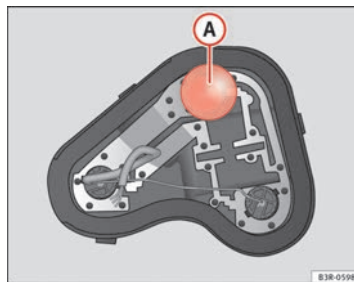
Fig. 210 Ubicación de la lámpara de incandescencia en el portalámparas. Ejemplo: Piloto posterior izquierdo en la aleta.
