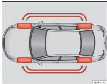
Fig. 175 Esquema para el cambio de ruedas
