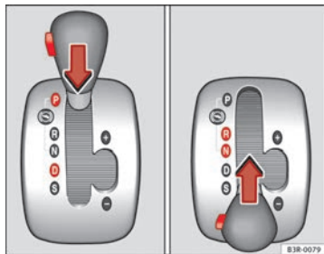
Fig. 145 Bloqueo de la palanca selectora
