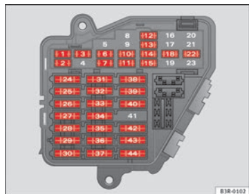
Fig. 186 Ilustración básica del portafusibles en la cubierta delantera izquierda del tablero de instrumentos: Fusibles (sin la tapa de los fusibles)
