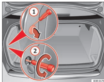
Fig. 206 Maletero: Posición del tornillo de fijación para la unidad de luz trasera
