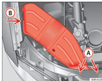
Fig. 218 Conducción de ventilación en el lado derecho del vehículo
