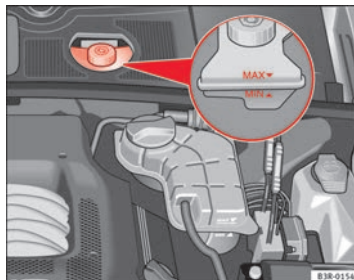
Fig. 189 Compartimento del motor: marcas en el depósito del líquido de frenos
