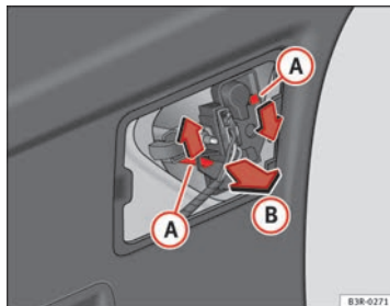
Fig. 235 Desmontar el portalámparas
