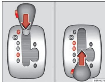
Fig. 160 Bloqueo de la palanca selectora
