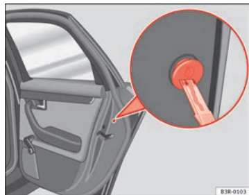
Fig. 73 Dispositivo de bloqueo de emergencia
