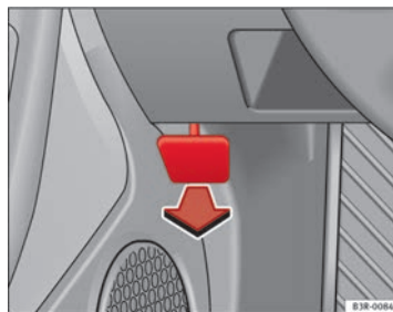
Fig. 179 Detalle de la zona reposapiés del lado del conductor: palanca para el desbloqueo del capó del motor. ►
