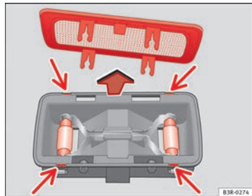
Fig. 240 Luz maletero
