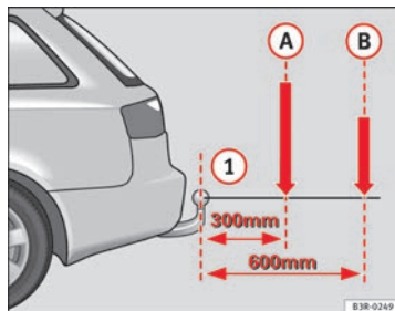
Fig. 165 Representación básica de la distribución de la carga de piezas accesorias y accesorios
