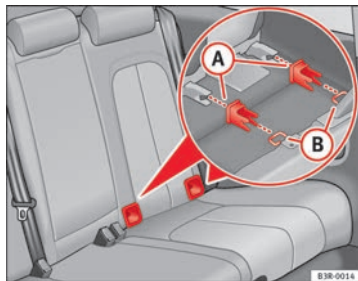
Fig. 33 Posición de los anclajes ISOFIX del asiento posterior lateral
