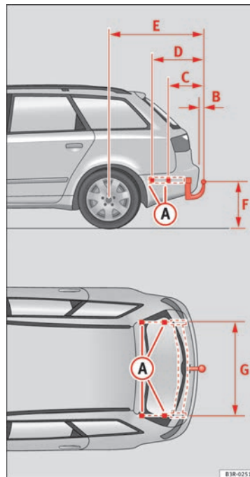
Fig. 176 Puntos de fijación del dispositivo de remolque
