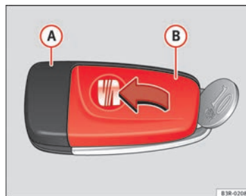
Fig. 70 Llave principal: Abrir la tapa
