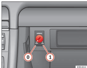
Fig. 28 En la guantera: conmutador con llave para activar y desactivar el airbag del acompañante
