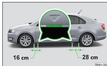
Fig. 241 Travesa de toma para el gato
