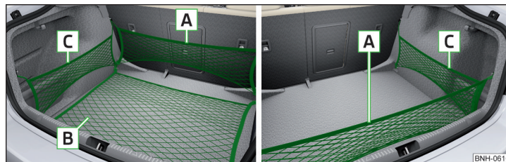
Fig. 100 Ejemplos de fijación para redes
