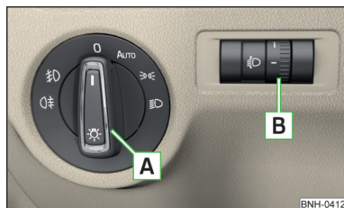
Fig. 52 Conmutador de luces y regulador giratorio para la regulación del alcance luminoso
