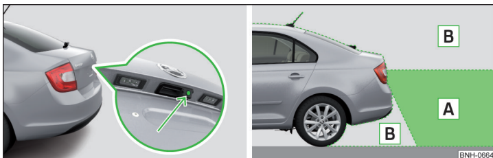
Fig. 197 Lugar de instalación de la cámara / área parpadeado detrás del vehículo
