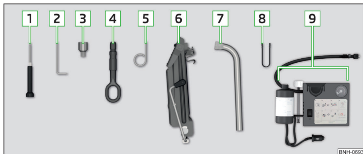
Fig. 236 Equipo de herramientas a bordo
