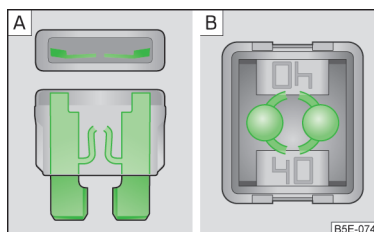
Fig. 256 Fusibles quemados
