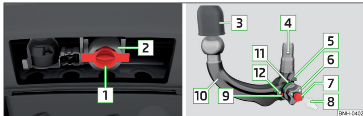
Fig. 210 Soporte del dispositivo de remolque / barra de cabeza esférica
