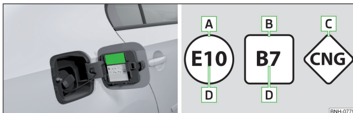
Fig. 222 Etiqueta con combustible prescrito / designación gráfica de los tipos de combustible
