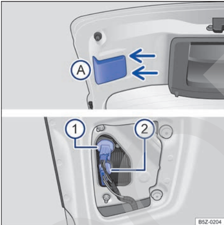
Fig. 149 Linterna trasera: (A) desmonte el cubierta y (1) y (2) desmonte las lámparas.
