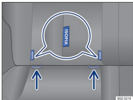
Fig. 19 En el asiento del vehículo: identificación de los puntos de anclaje inferiores de asientos para niños.
