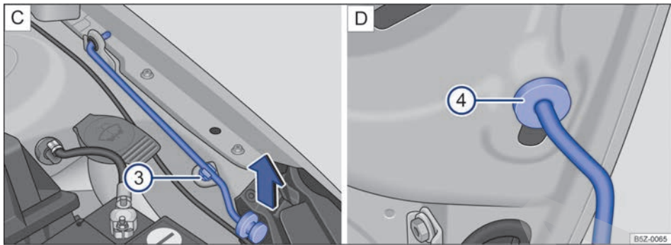
Fig. 168 C: varilla de sujeción de la tapa del compartimento del motor (3). D: tapa del compartimento del motor protegida con la varilla de sujeción de la tapa (4).
