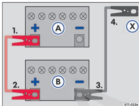
Fig. 160 Esquema para la conexión de los cables auxiliares de arranque: batería del vehículo descargada (A) y batería del vehículo que provee la corriente (B).
