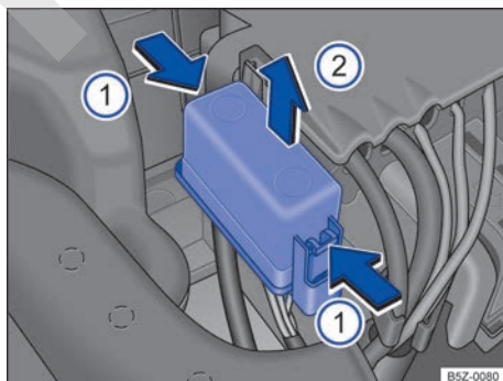
Fig. 154 En el compartimento del motor: cobertura de la caja de fusibles.
