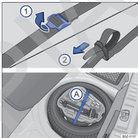
Fig. 137 En el maletero: cinta de fijación de la caja de herramientas y caja de herramientas de a bordo.
