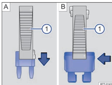
Fig. 158 Quitar o instalar un fusible con la garra de la pinza de plástico ①.
