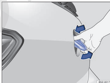
Fig. 61 Abrir la tapa trasera por afuera.
