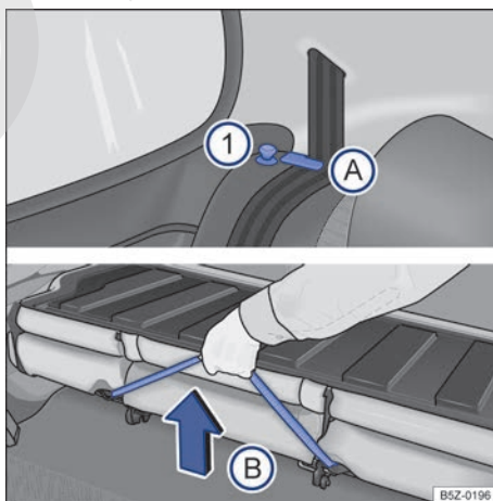
Fig. 71 Asiento trasero: pasadores de desbloqueo ①; posicionador para las bandas de los cinturones A; manija para desbloqueo del conjunto del piso B.
