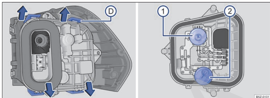
Fig. 148 Linterna trasera: D desmontar el portalámparas y 1 y 2 desmontar las lámparas incandescentes.
