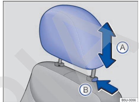
Fig. 75 Desmonte el apoyacabezas delantero.
