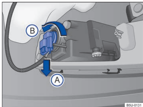
Fig. 144 Detrás del parachoques delantero: acceso a la lámpara incandescente del farol de neblina.
