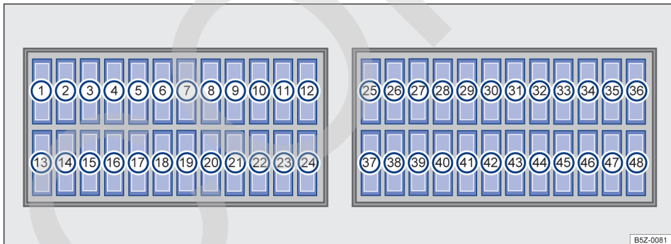
Fig. 155 Caja de fusibles.
