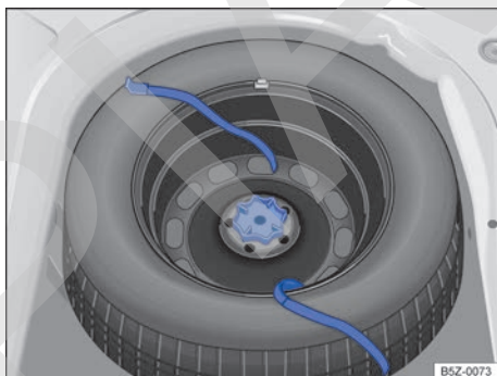
Fig. 181 En el maletero: manivela para fijación de la rueda de emergencia.
