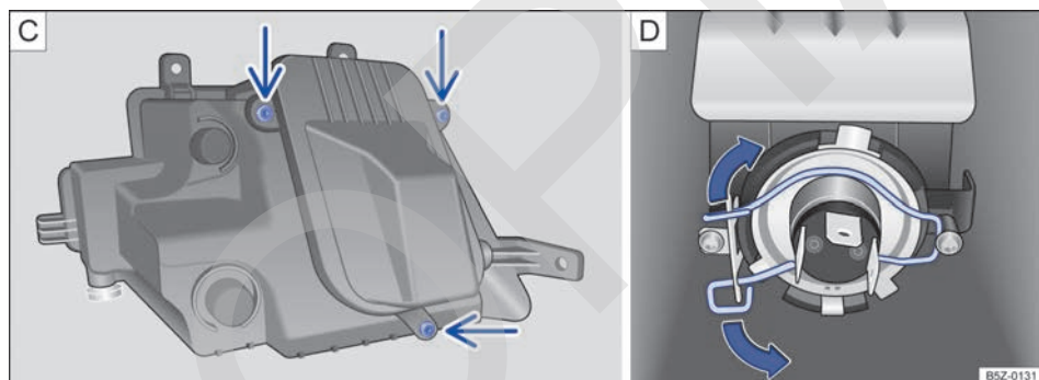
Fig. 146 En el parachoques delantero: Ⓒ retirar los tornillos de la cubierta de la bombilla y Ⓓ bombilla del faro de neblina.
