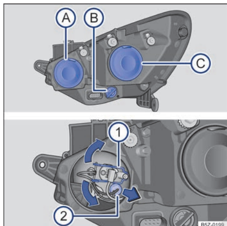
Fig. 142 En el compartimento del motor: vista trasera del farol delantero derecho con cubierta de goma (izquierda): A farol alto y luz de posición, B indicadores de dirección y C farol bajo. Vista trasera del farol delantero derecho sin cubierta de goma (derecha): 1 farol alto, 2 luz de posición.
