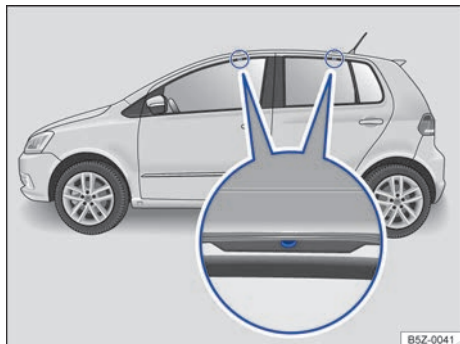
Fig. 132 Puntos de fijación de los soportes básicos del portaequipaje de techo (ambos lados)
