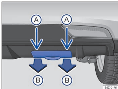
Fig. 166 En el paragolpes trasero a la derecha: argolla de remolque trasera - paragolpes con cubierta desmontable.
