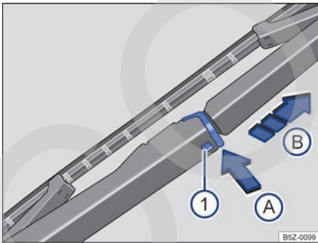
Fig. 141 Sustituir la escobilla del limpiaviento.
