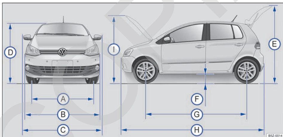
Fig. 193 Dimensiones.
