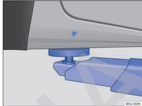
Fig. 188 Puntos de apoyo delanteros para la suspensión con plataforma elevadora o con gato.
