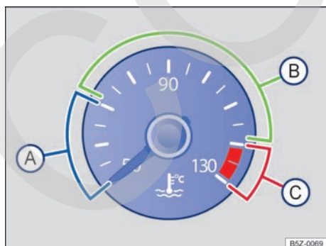
Fig. 40 Indicador de temperatura del líquido de refrigeración del motor en el panel de instrumentos: A zona fría; B zona normal; C zona de alerta.
