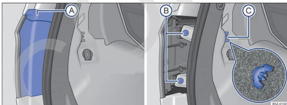
Fig. 147 Lateralmente en el maletero: A ) desmonte la cubierta, B ) retire los dos tornillos y C ) retire el tornillo mariposa (fragmento ampliado). ▶
