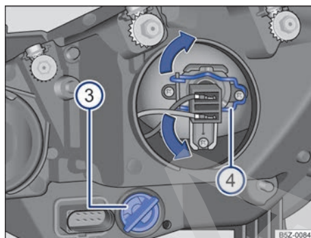
Fig. 143 En el compartimento del motor: vista trasera del farol delantero derecho sin cubierta de goma: 3 indicadores de dirección y 4 farol bajo.
