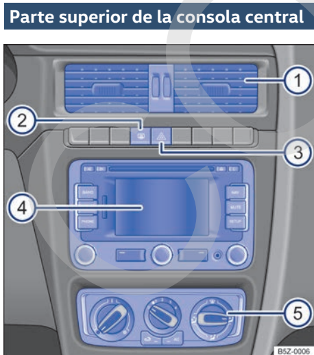
Fig. 32 Vista general de la parte superior de la consola central.
