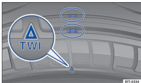
Fig. 180 Perfil del neumático: indicadores de desgaste.
