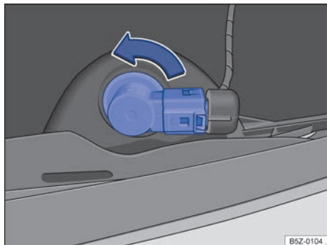
Fig. 150 Detrás del paragolpes trasero: acceso a la lámpara incandescente de la linterna de neblina (sólo lado izquierdo).
