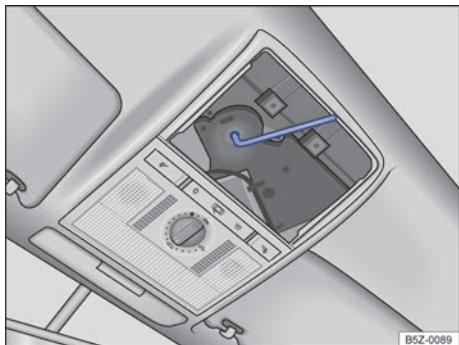
Fig. 67 Tornillo hexagonal para cierre del techo solar.
