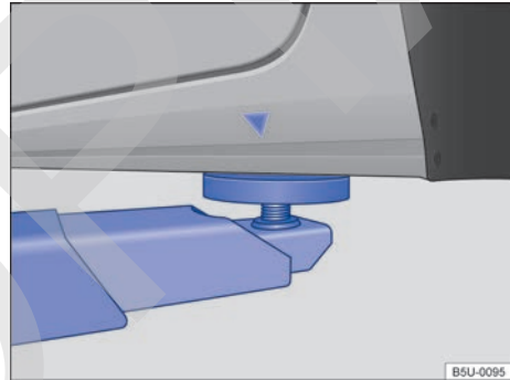
Fig. 189 Puntos de apoyo traseros para la suspensión con plataforma elevadora o con gato.
