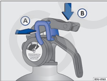
Fig. 26 Secuencia de uso del extintor de incendio.
