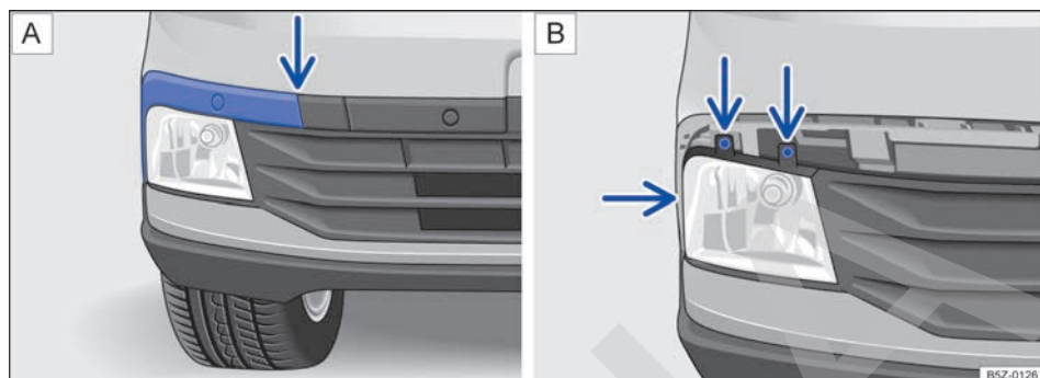
Fig. 145 En el parachoques delantero: Ⓐ desinstalar la moldura del faro de neblina y Ⓑ retirar los tornillos del faro de neblina.
